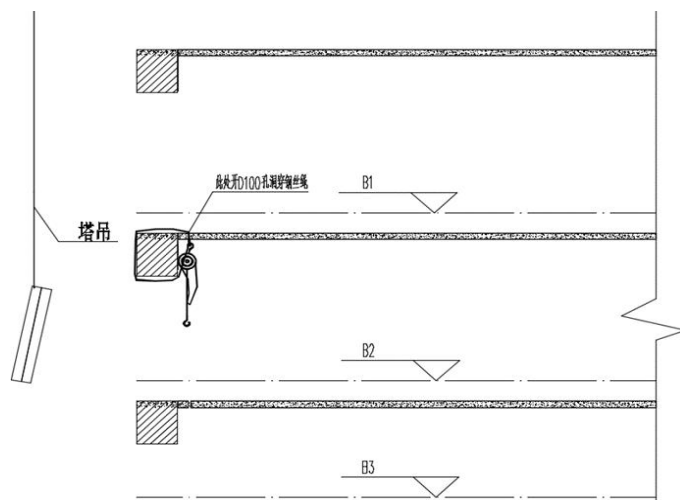
图 5.2.5-3 钢梁吊装示意图
