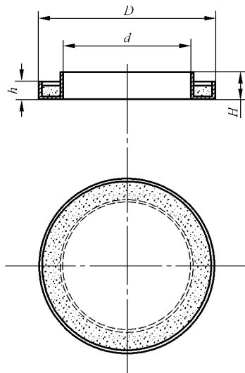
图1 环形吸气剂示意图
