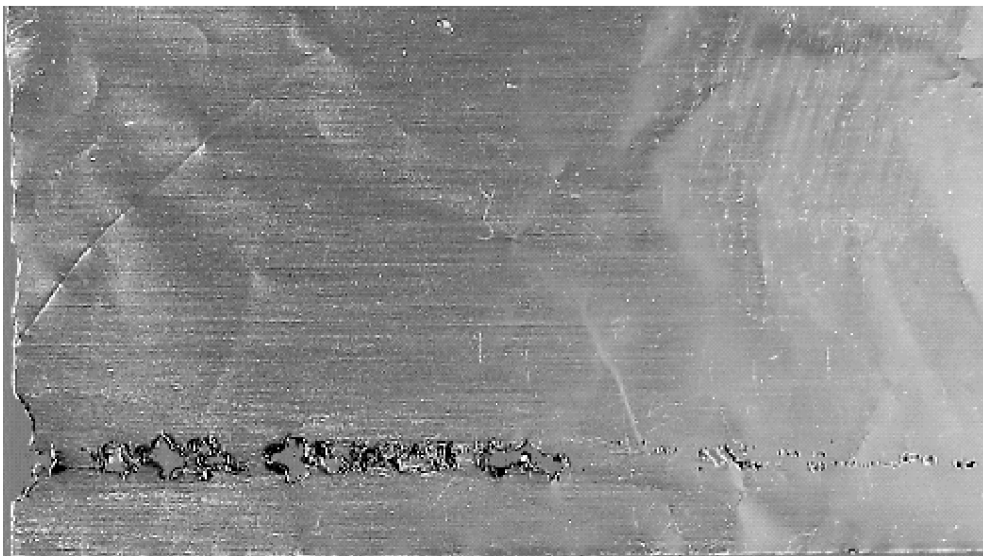
图1 非金属压入
