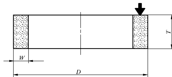
图 1 2 型砂轮
