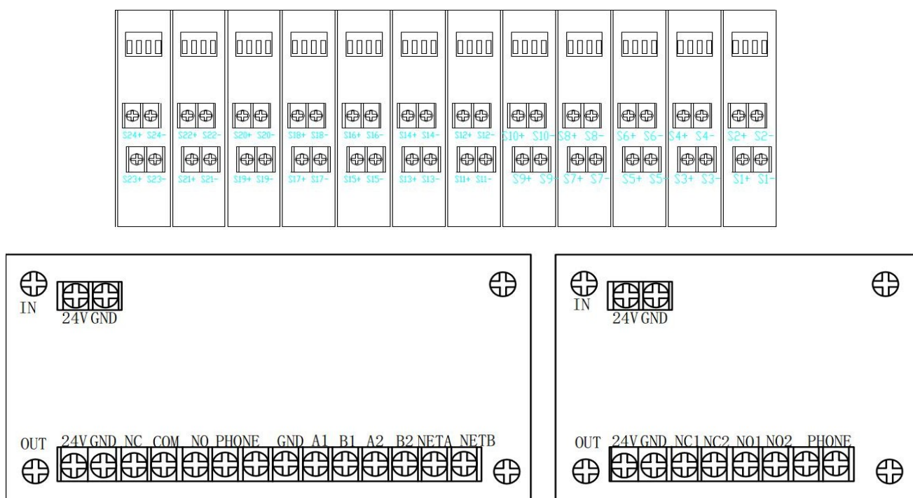
图 3 控制器接线盘及接线端子位置图
