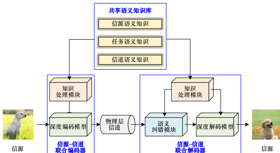
图 8 语义知识库使能的信源-信道联合编码框架
