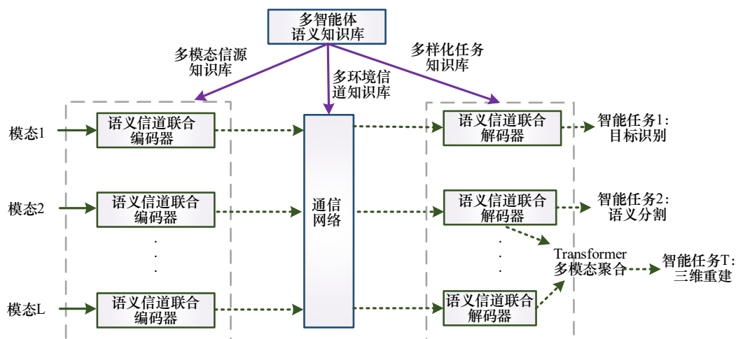
图 6 基于多智能体知识库的语义传输框架示意图
