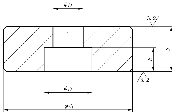
图 1 垫圈
