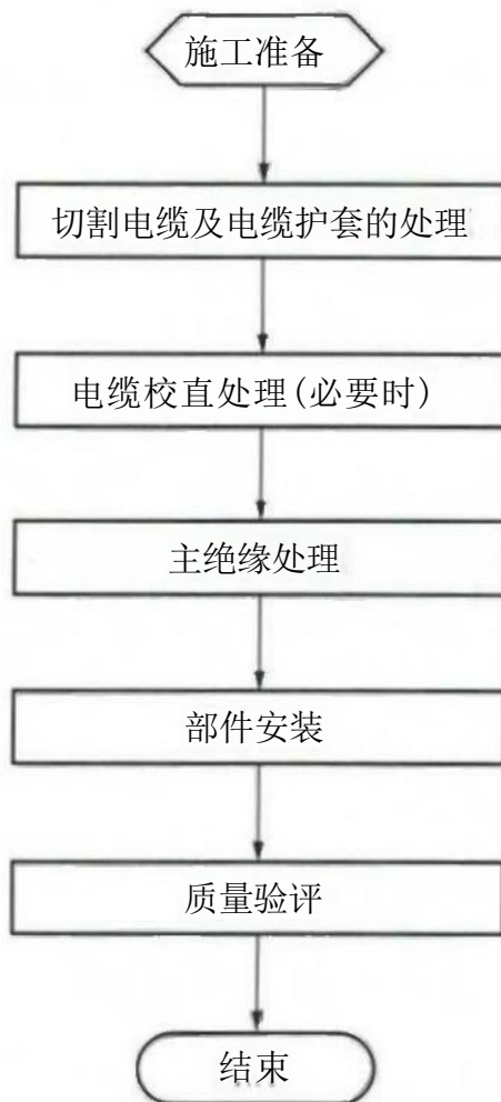
图4.0.1 电缆附件安装工艺流程图
