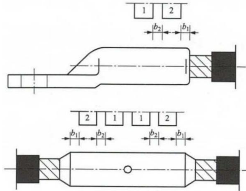
图5.5.4 压接时的压接顺序和压痕距离
