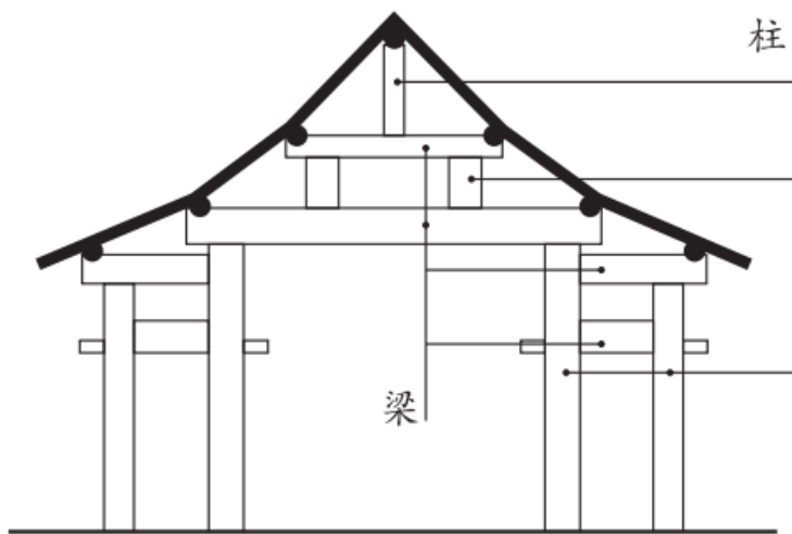
中国古建筑大木构架剖面示意图
