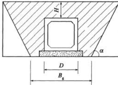
图 5.2.3 箱涵与地形关系示意图
