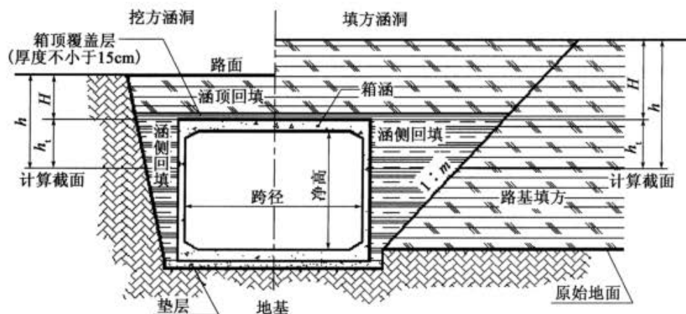
图 3.0.4 箱涵典型横断面示意图
