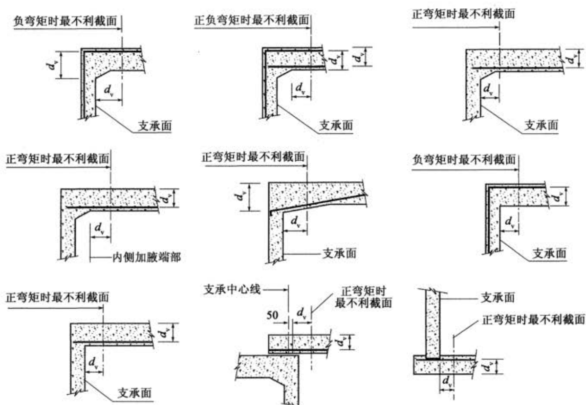
图 5-1 箱涵抗剪承载力验算最不利截面示意
