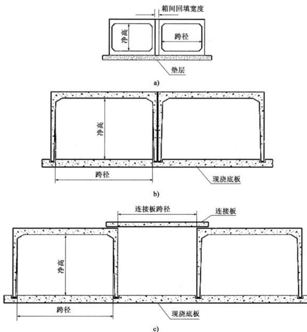
图 3.0.7 多室箱涵横断面布置示意图
