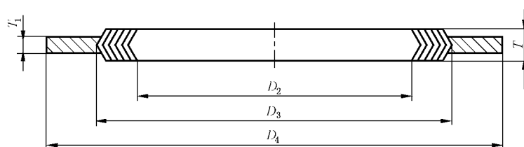
图 1 带定位环型缠绕式垫片
