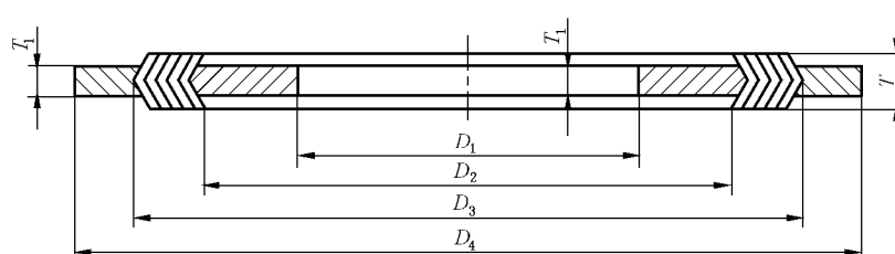
图 2 带内环和定位环型缠绕式垫片
