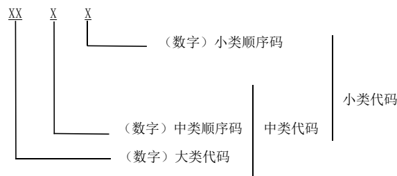
图2 代码结构
