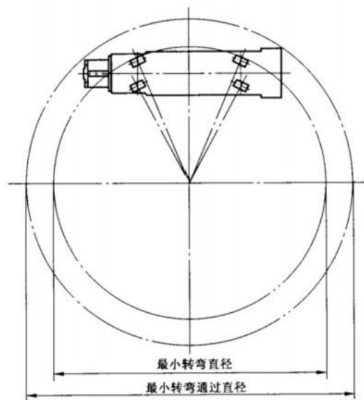
图 1 最小转弯直径图
