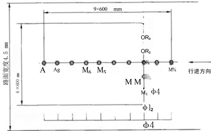
图 2 温度布点测试图
