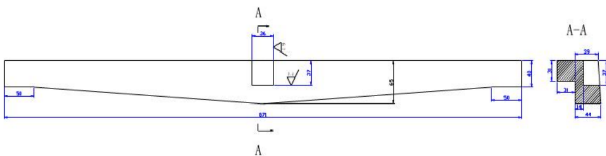
图 2.11 篦条示意图
