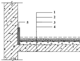
图 5.3.1 石膏复合材料建筑楼板隔声保温系统基本构造
