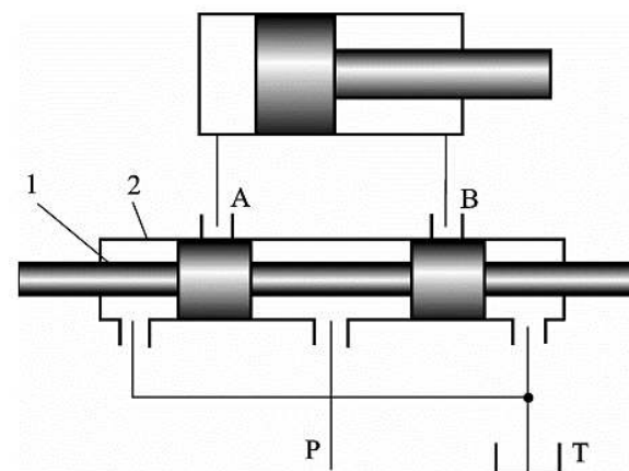
1-阀芯；2-阀体
