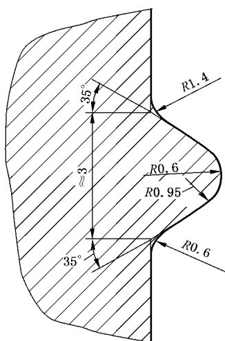
图 1 铣刀轮廓
