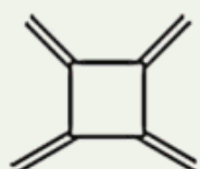
[4]轴烯 (b)
