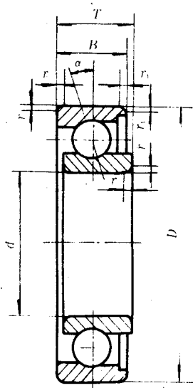
图 1 分离型角接触球轴承 S70000 型( \alpha = 15^\circ )
