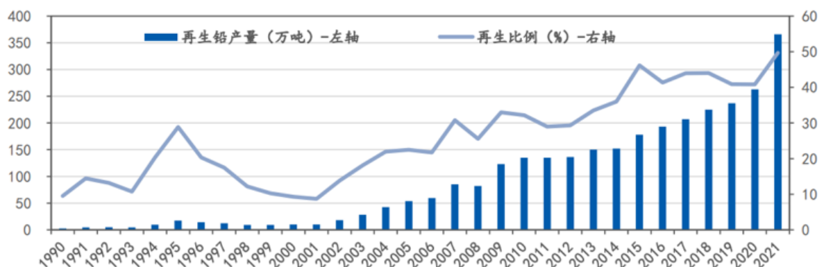
图 12：再生铅产量
