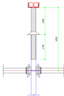
1.2m水平杆
