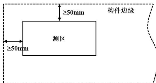
图6 测区范围选择示意图
