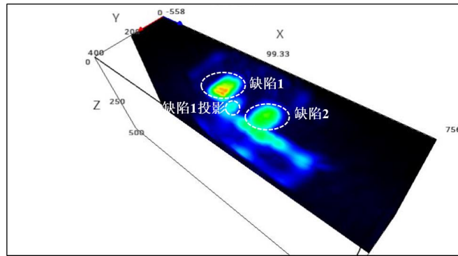
图 10 体扫描模式下缺陷的确定示意图
