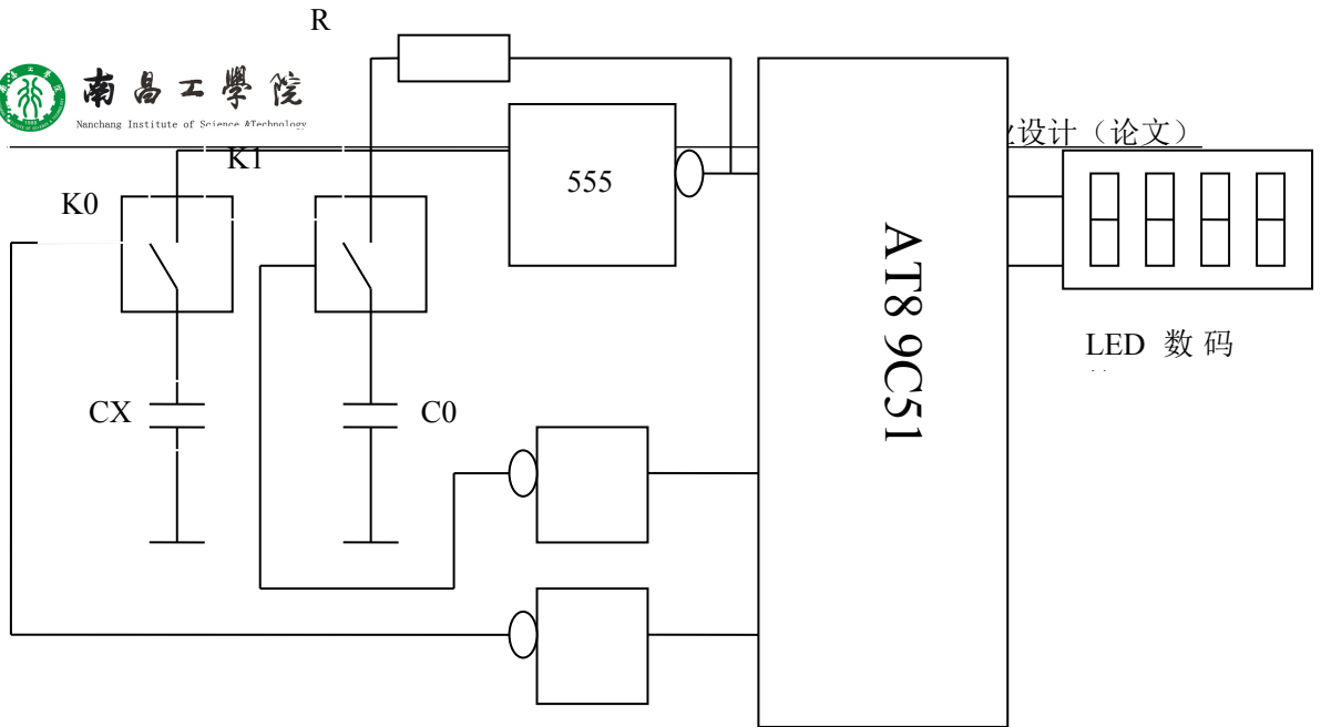
图 1 电容测量原理图
