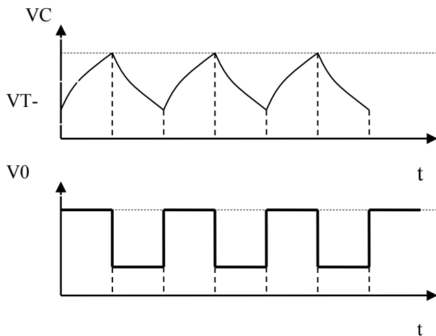
图 2 震荡波形图
