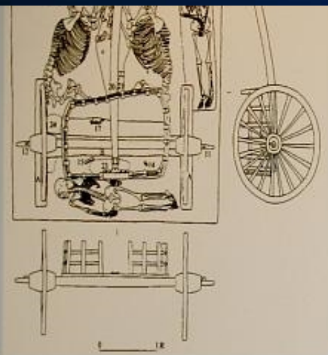
车马坑 M 52平面图、车子侧视图、衡后视图
