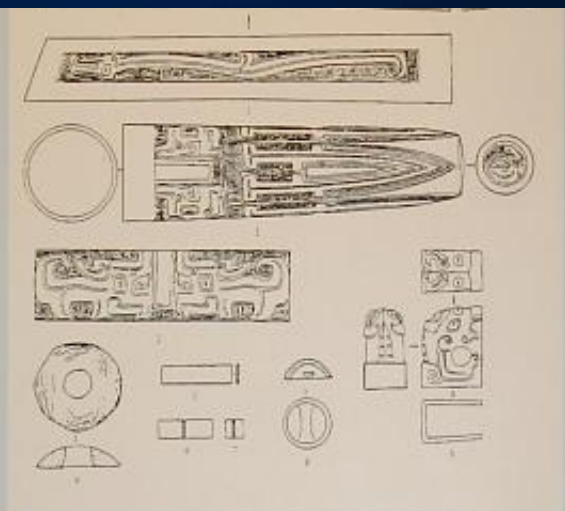
车马坑 M 52出土铜杆头、轭和蚌环等
