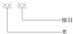
图 1 代码结构图
