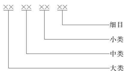
图 1 代码结构图
