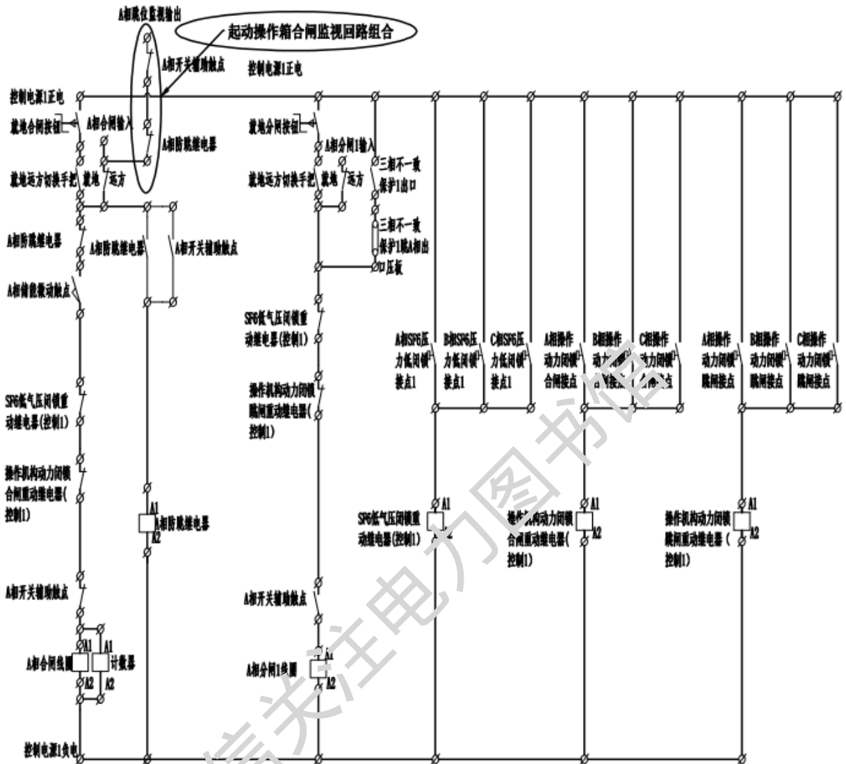
图 3 防跳回路连接示意图
