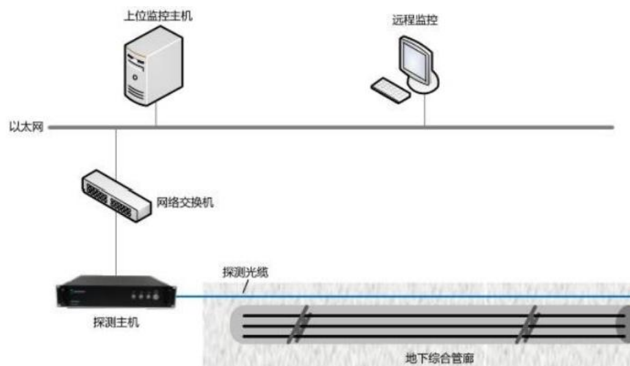
图 1 3 防外破监测系统
