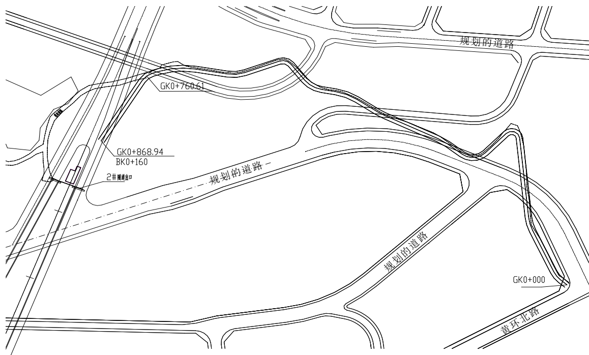
图 1-5 3#路基施工便道平面布置图
