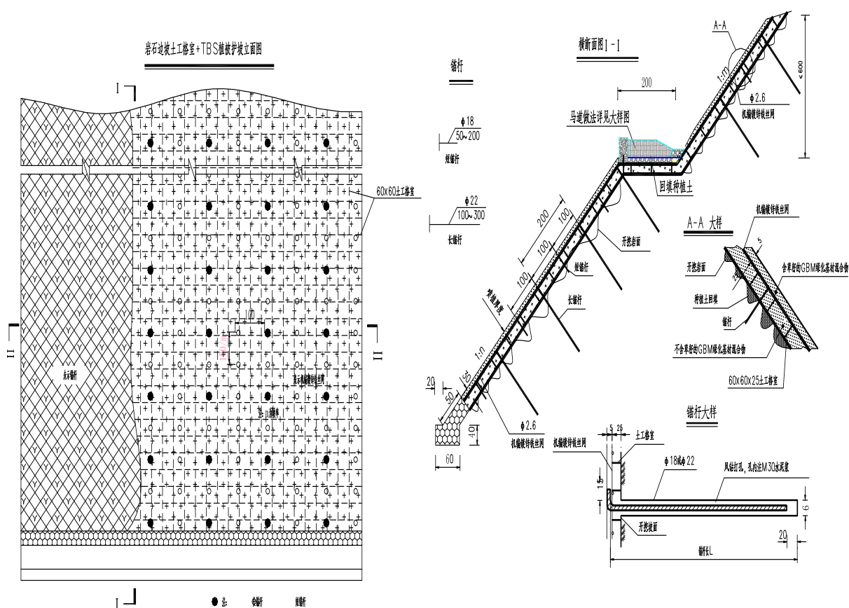
图 4-8 土工格室大样图
