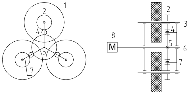
三角行星构造原理示意图
