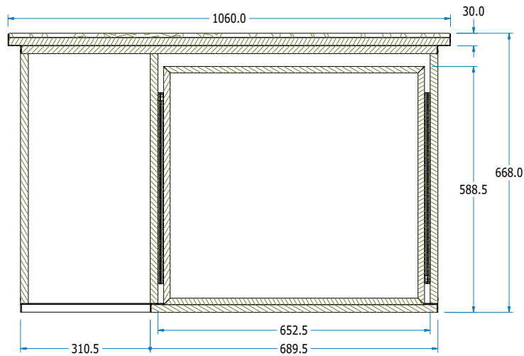
SECTION C-C SCALE 0.11 : 1
