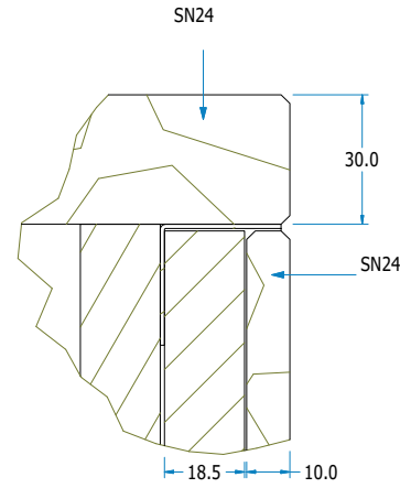
DETAIL B SCALE 0.22 : 0.3
