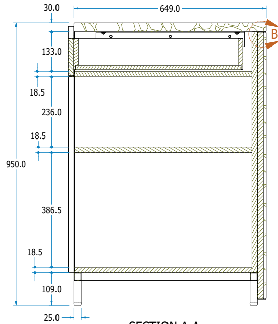
SECTION A-A SCALE 0.11 : 1
