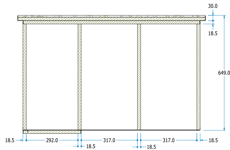
SECTION D-D SCALE 0.11 : 1
