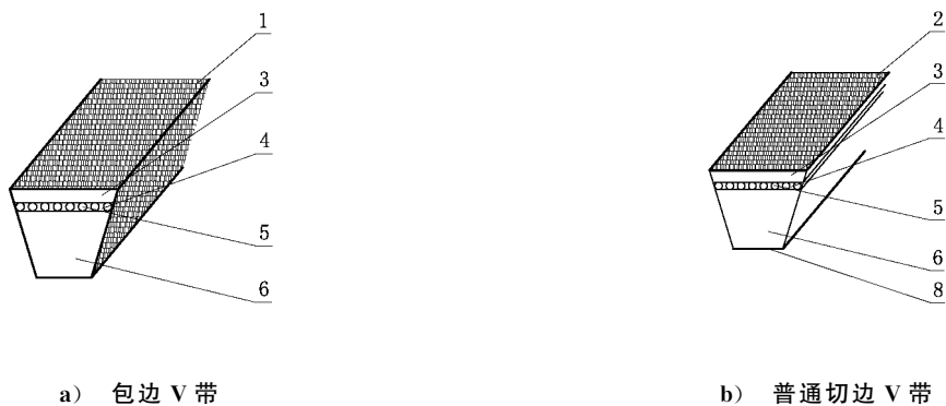
图 1 V 带结构示意图
