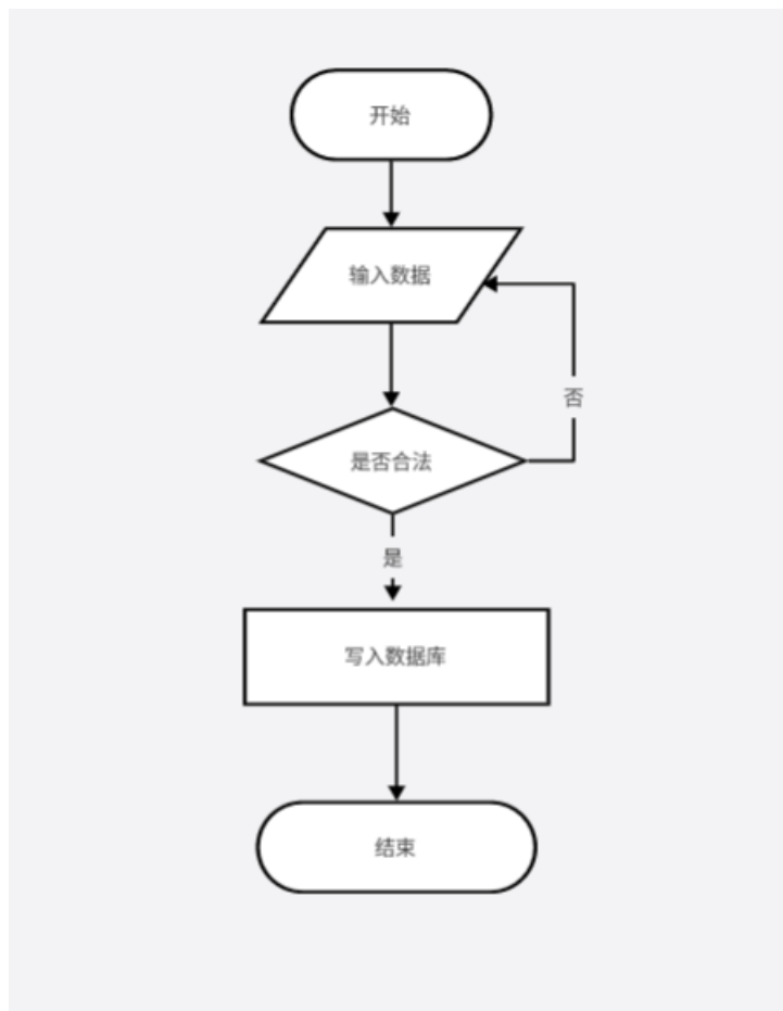
图 3.3 添加信息流程图
