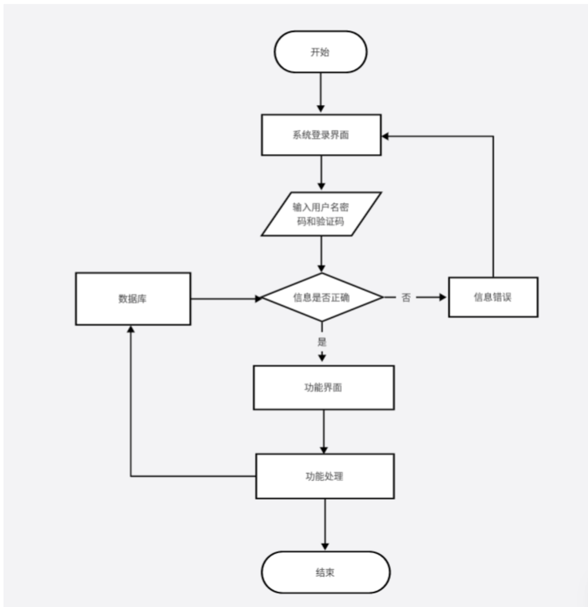
图 3.2 系统操作流程
