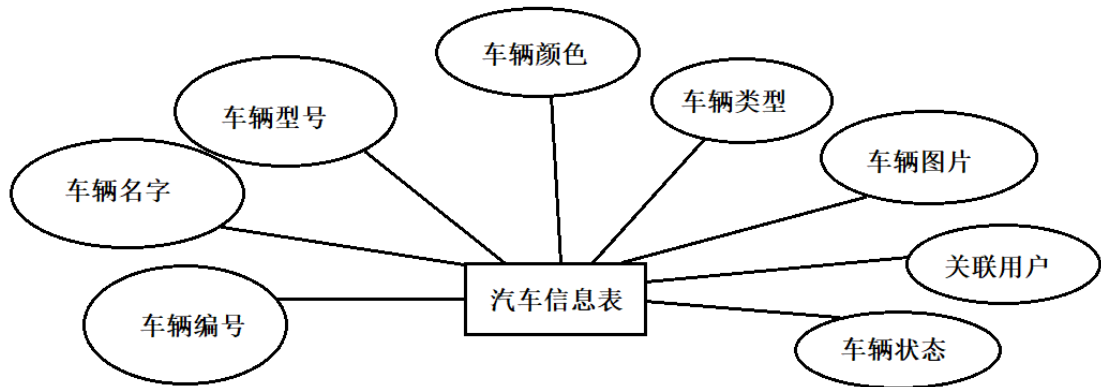
图 4.4 汽车信息表实体图
