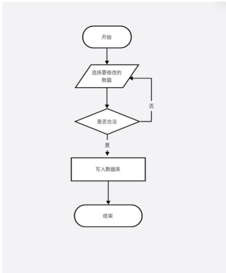
图 3.4 修改信息流程图
