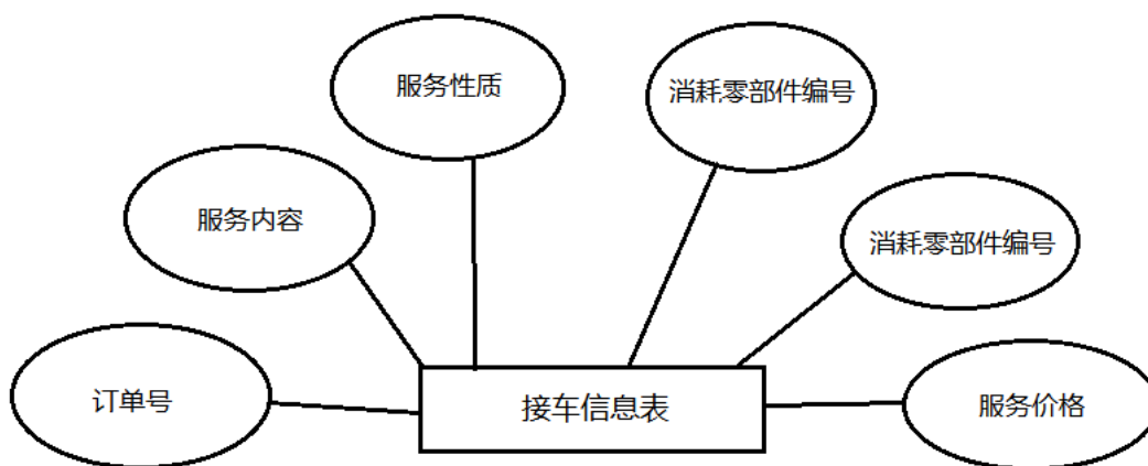
图 4.9 维修保养服务信息表实体图
