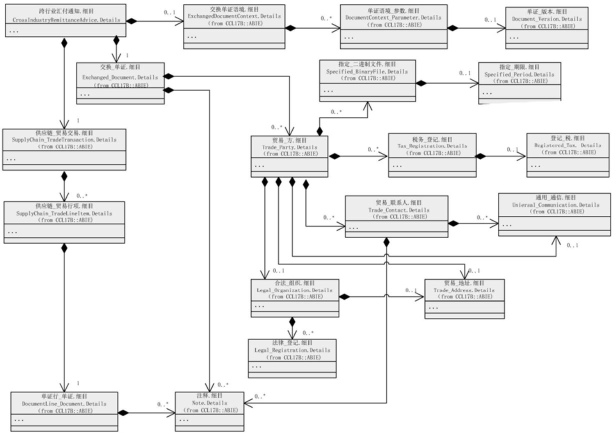
图 2 交换单证、交换单证语境和单证行文件
