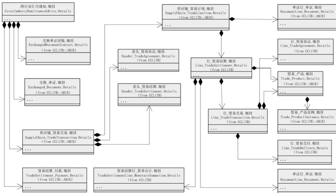
图 1 跨行业汇付通知的概念数据模型
