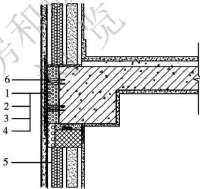
图5.3.2-2 自保温墙体与混凝土梁连接部位构造
