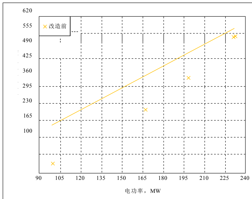
图 01 供热抽汽流量与电功率的关系曲线
