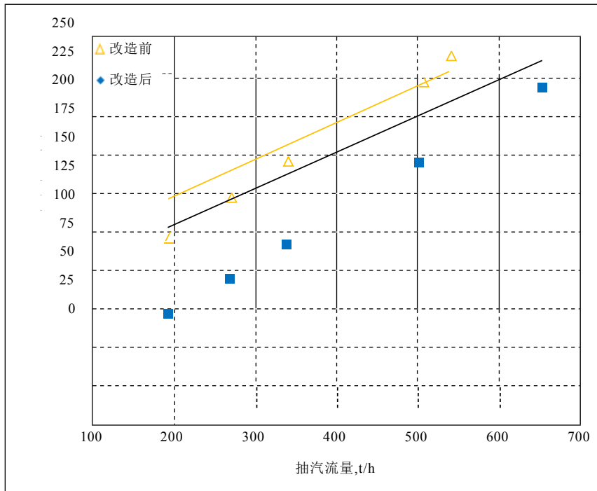
图 03 相同抽汽流量条件下，改造前后机组供热特性对比
