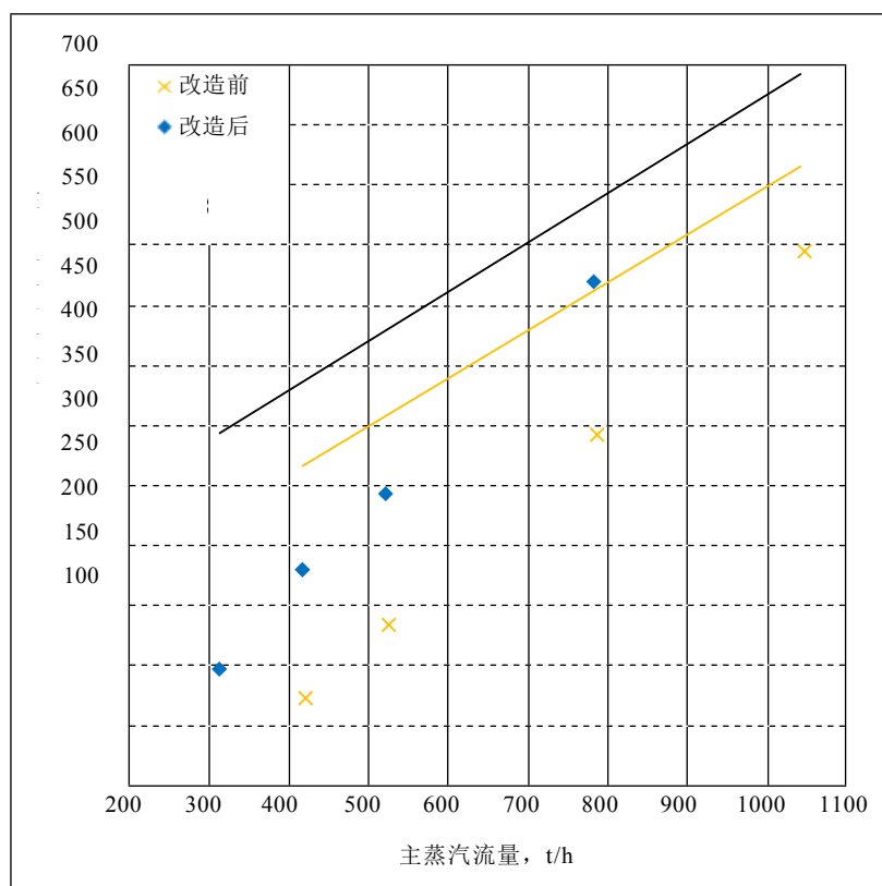
图 02 主蒸汽流量与供热抽汽流量的关系曲线
