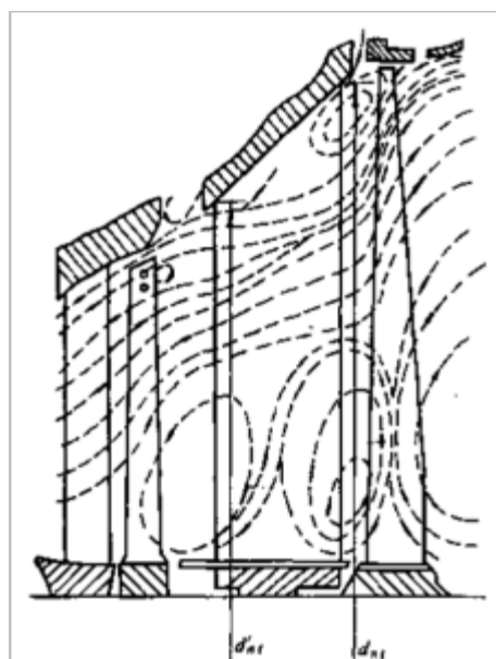
图 06 某汽轮机末级叶片小容积流量工况流线示意图
