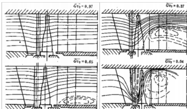
图 05 容积流量减小时，低压缸末级叶片内流动状态变化示意图
