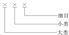
图 1 代码结构图
