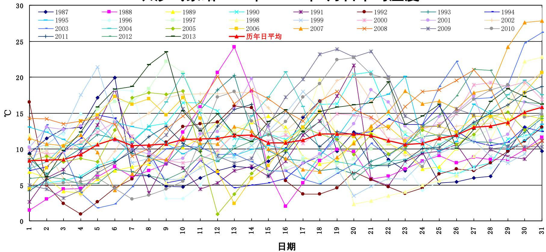
长沙气象站1987年~2013年3月日平均温度
