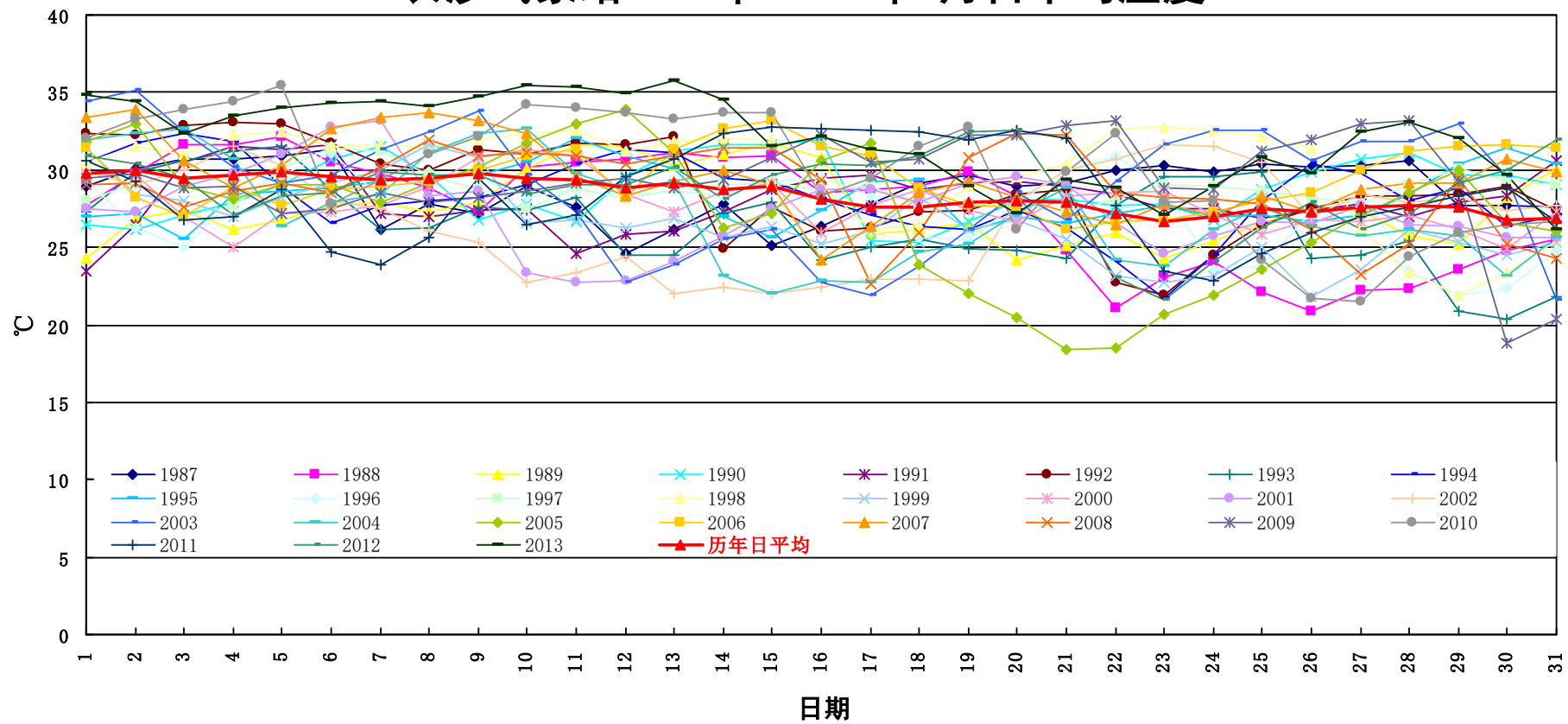
长沙气象站1987年~2013年8月日平均温度
