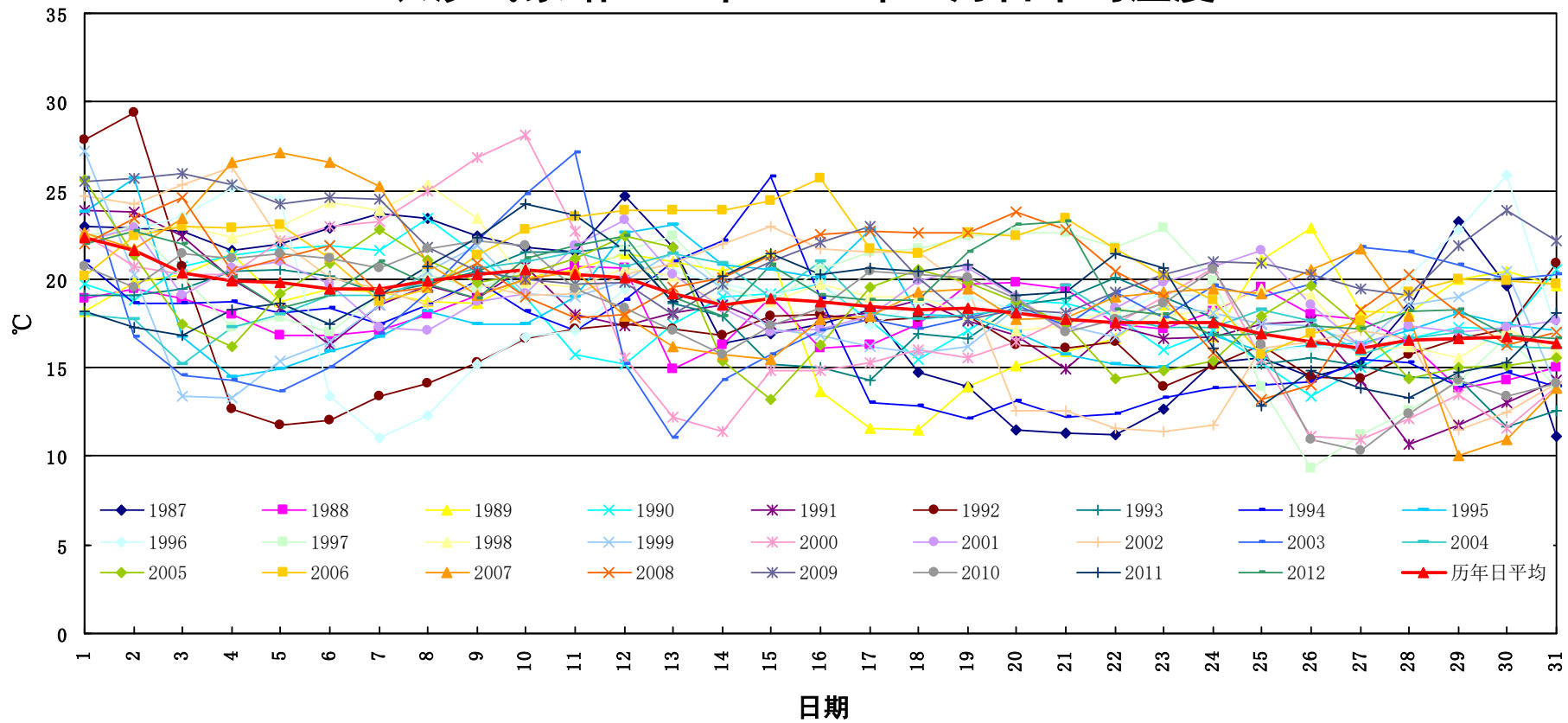
长沙气象站1987年~2012年10月日平均温度
