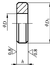
图 1 推板垫圈
