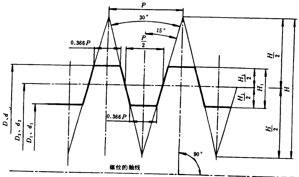
图1 基本牙型
