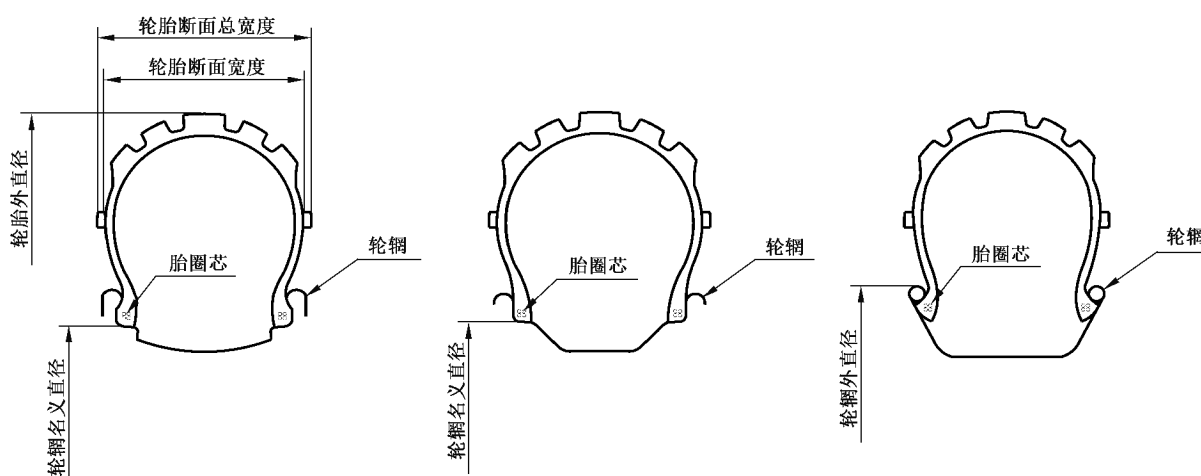
图 1 钩直边(CT)轮胎断面
