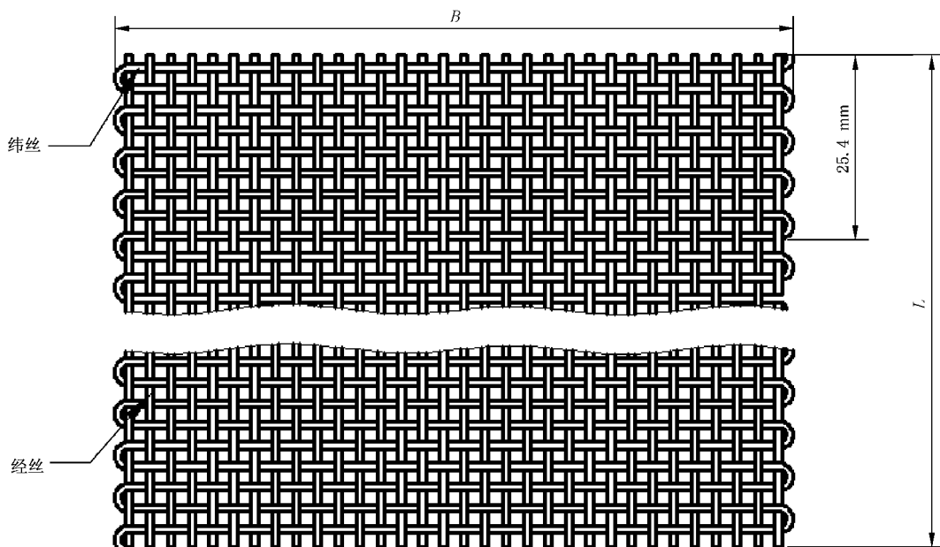
图1 垫网结构简图
