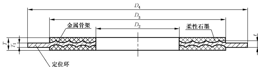
图 2 带定位环型
