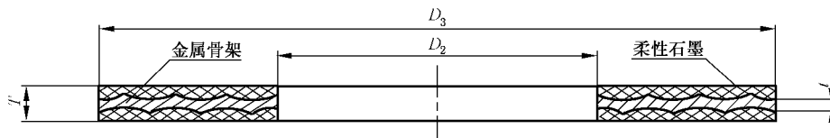
图 1 基本型
