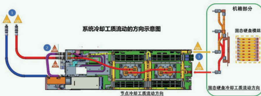
图3. 2U四节点全液冷服务器串联流路
