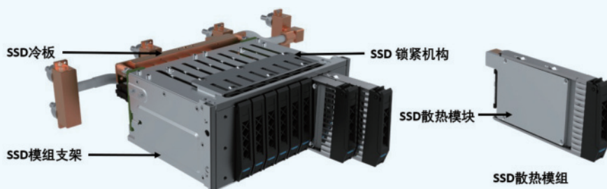
图6. 创新的固态硬盘液冷方案
