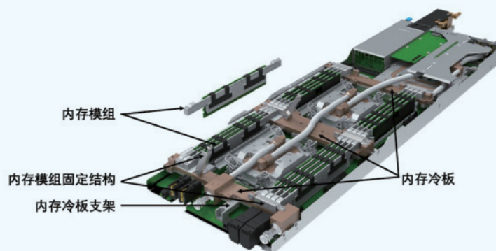
图5. 枕木散热器液冷方案
