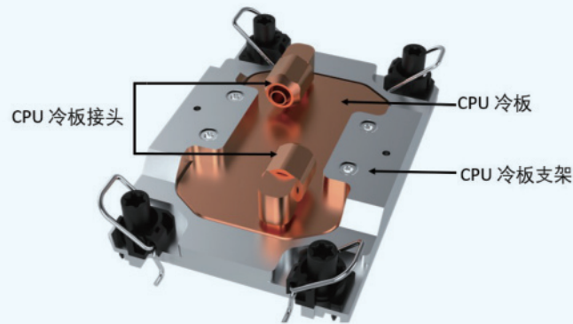
图4. CPU冷板模组
