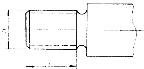
图2 外螺纹（带肩）
