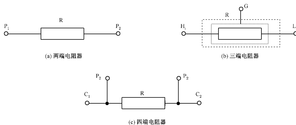
图 1 直流标准电阻器结构图
