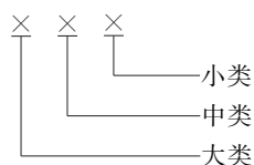
图 1 代码结构图
