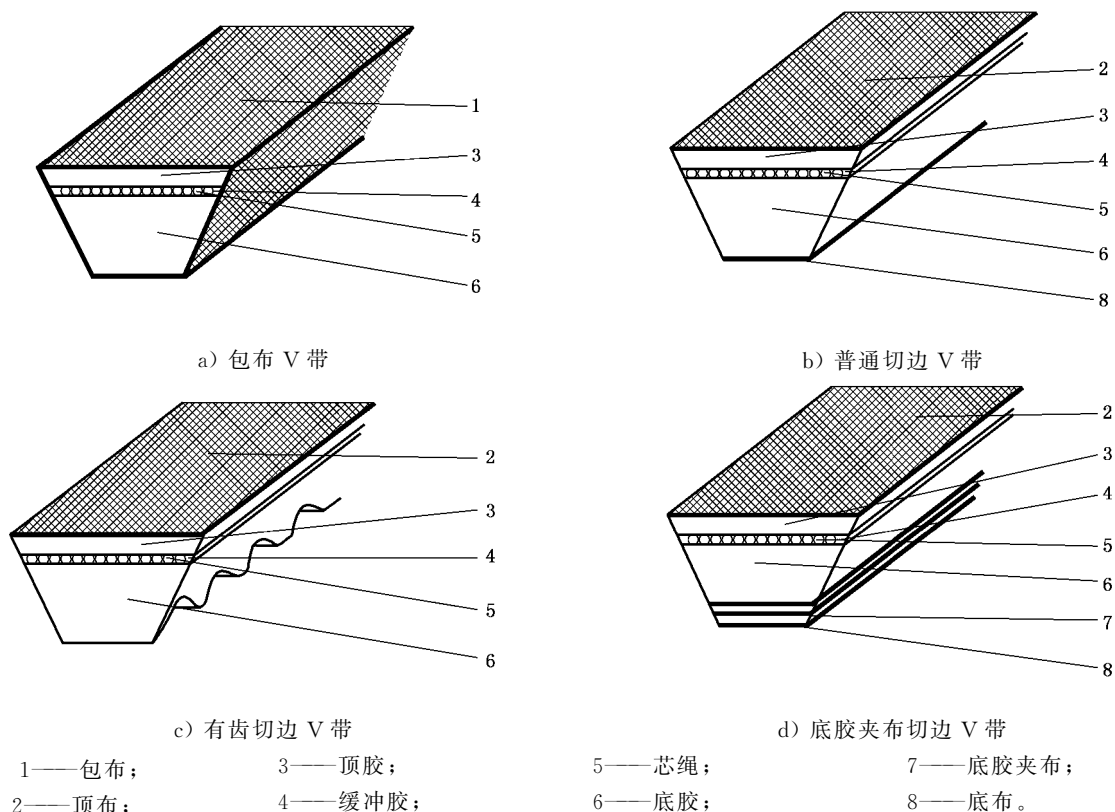
图 1 V 带的结构
