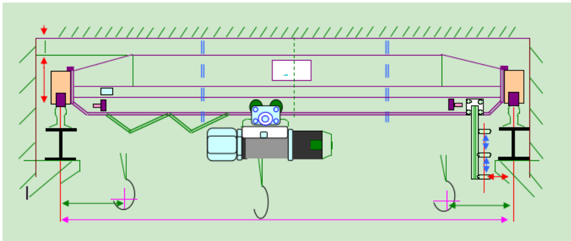
地操外形总图
