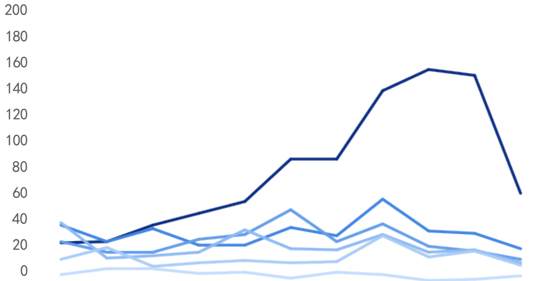
2013-2023年全球电动牙刷有效公开专利数量
